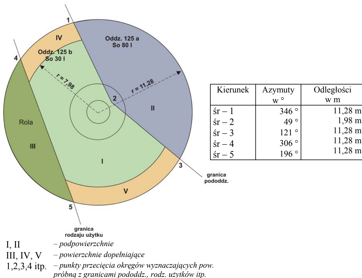
Rys. 7. Przykłady szkicu powierzchni próbnej
