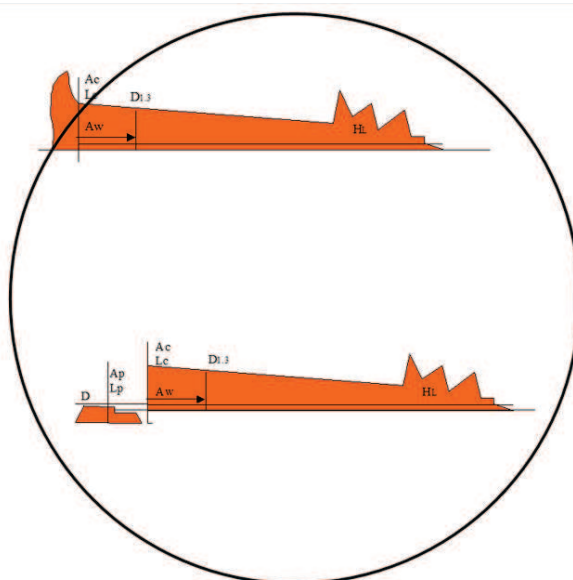
Rys. 16. Sposób pomiaru drzew ściętych i wyrwconych
