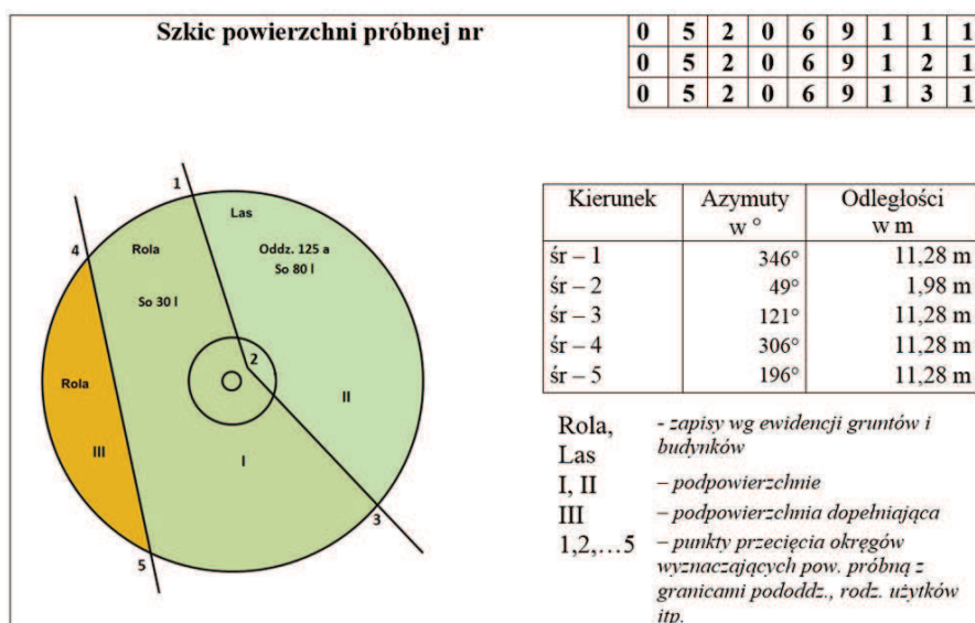
Rys. 8. Przykład szkicu powierzchni próbnej
