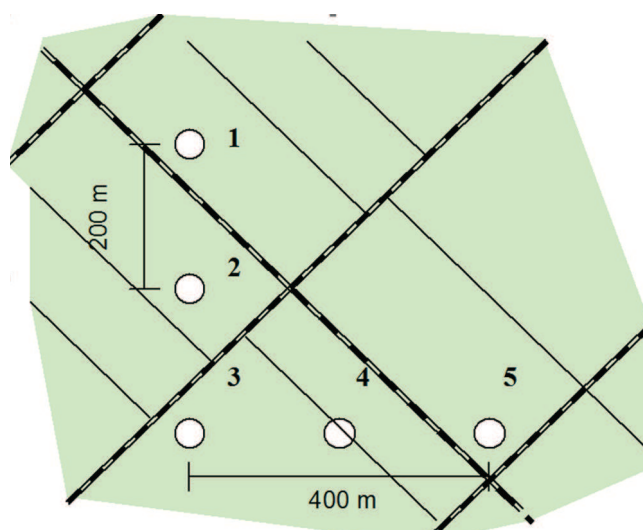
Rys. 2. Układ traktu na tle przykładowego podziału powierzchniowego
