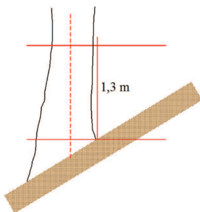
Rys. 11. Sposób ustalania wysokości 1,3 m w terenie nachylonym
